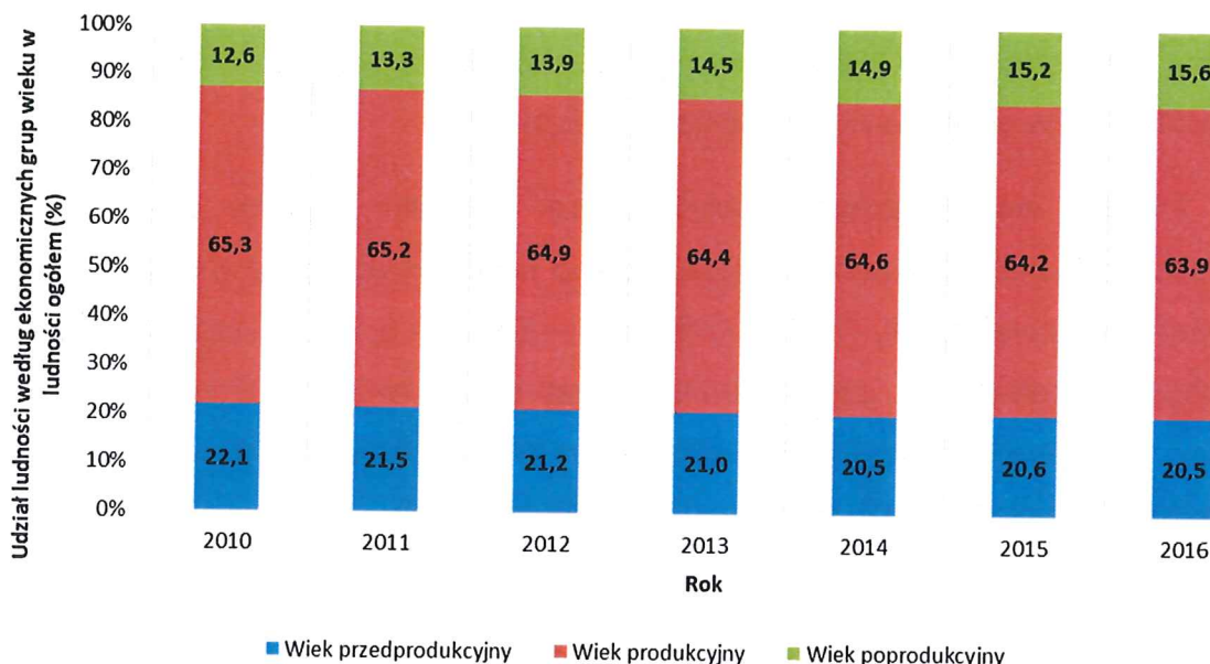
Wykres 3: Udział ludności według ekonomicznych grup wieku w ludności Gminy ogółem (%) w latach 2010 – 2016
